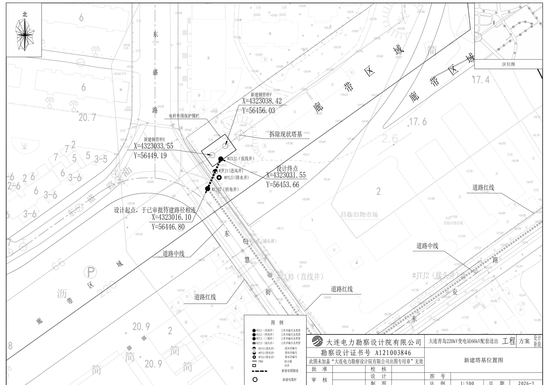
新建塔基位置图：
