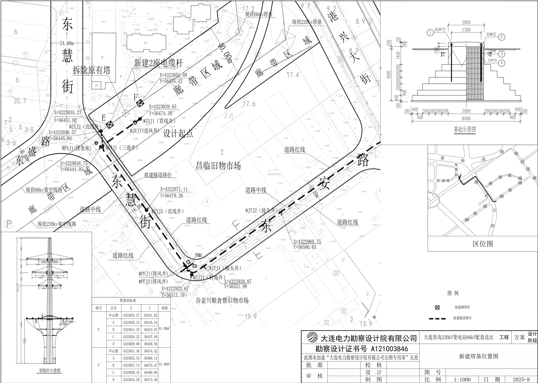
新建塔基位置图：
